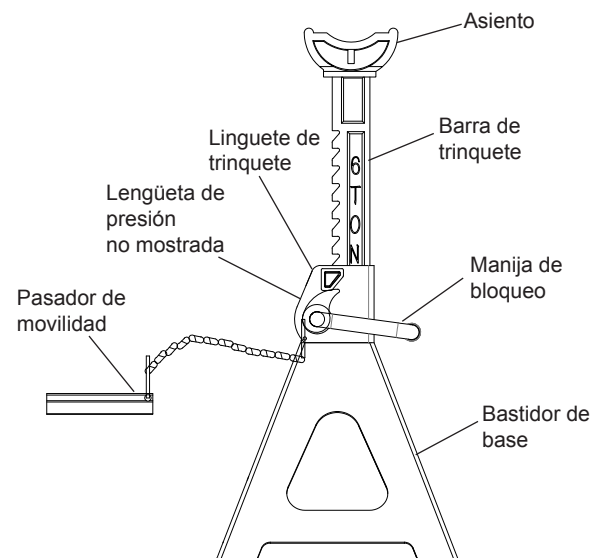
Figura 1: Nomenclatura habitual de un soporte de gato
